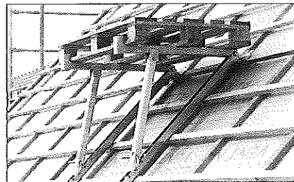
Echafaudage de versant en alu DS 680 A
